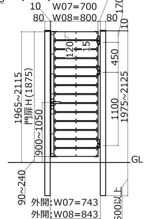
14段 すきま15mm (T-20)
