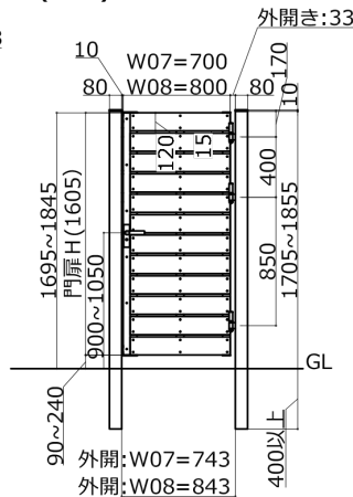
12段 すきま5mm (T-18)
