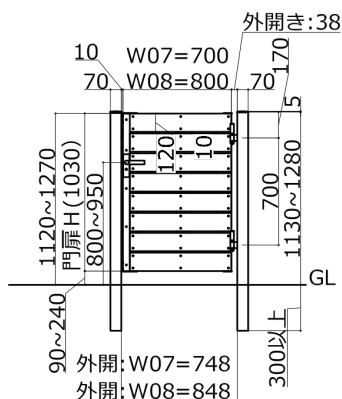
12段 すきま10mm (T-17)
