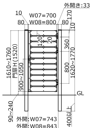
11段 すきま20mm (T-17)
