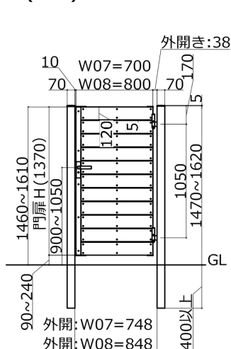
15段 すきま5mm (T-20)
