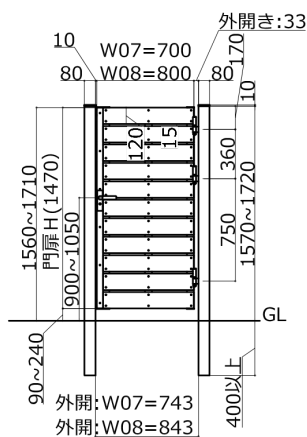
11段 すきま15mm (T-16)
