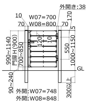
11段 すきま10mm (T-16)
