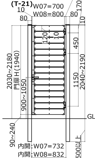
15段 すきま10mm 外開き:33 (T-21) W07=700 \frac{700}{20}
