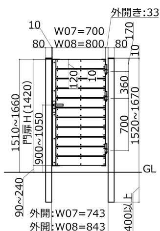
15段 すきま10mm 外開き:33 (T-21) W07=700 \frac{700}{20}
