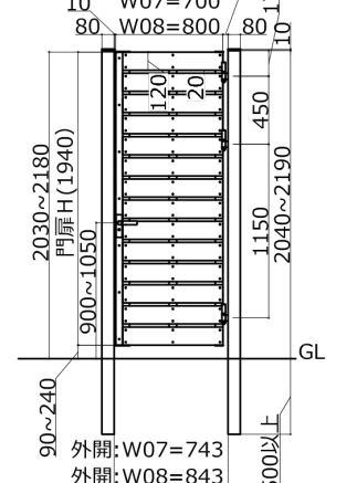
14段 すきま20mm (T-21)
