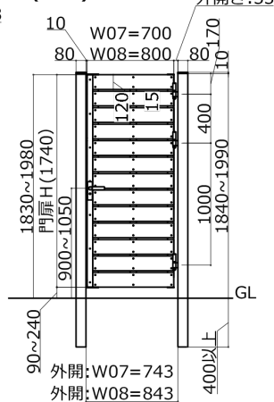
13段 すきま15mm (T-19)
