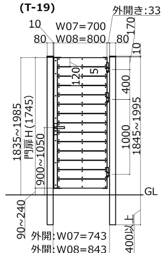
14段 すきま5mm (T-19)
