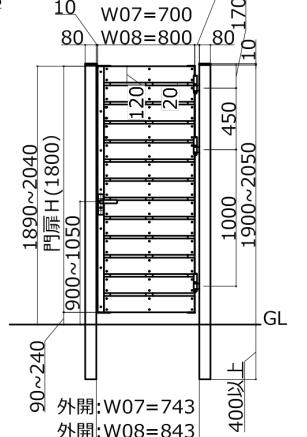
13段 すきま20mm (T-19)
