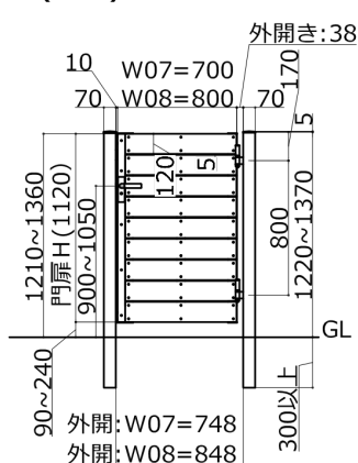
13段 すきま5mm (T-18)
