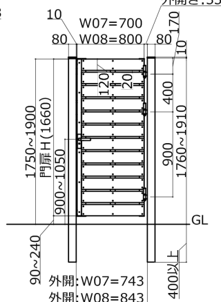
12段 すきま20mm (T-18)
