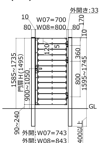
16段 すきま5mm (T-21)
