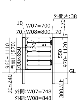
11段 すきま5mm (T-15)
