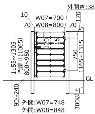
12段 すきま5mm (T-18)
